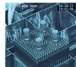
< 상단고정체 분해 >
