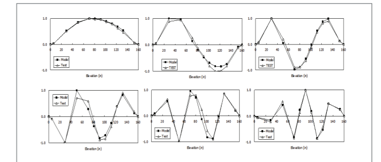
< 핵연료 동특성에 대한 DYTRAC 단순모델 검증 >
