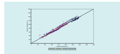
< ROPER 코드의 핵연료중심선 온도 측정치 및 예측치 비교 >
