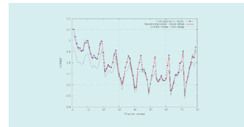
< THALES DNBR 예측 성능 >
