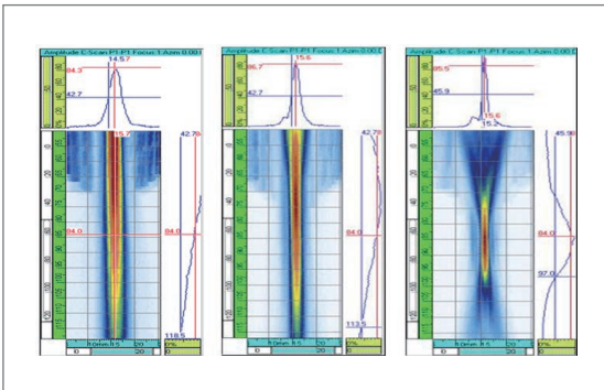
< 빔 시뮬레이션을 이용한 성능검증 >
