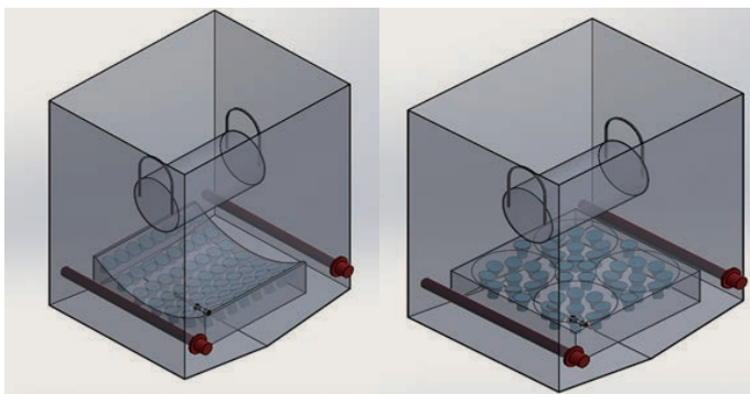
< 단계별 초음파 제염시스템 개략도 >
